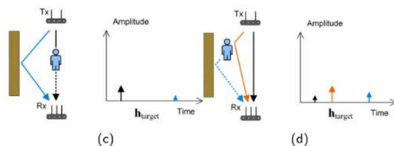
รูปที่ 2.6 แผนภาพช่องสัญญาณเป้าหมาย ในลักษณะสัญญาณตกค้างเชิงผลต่าง กรณีเป้าหมายบดบัง พารสายตรงและบดบังพารสะท้อน [2]
