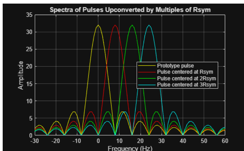
รูปที่ 2.4 กราฟโดเมนความถี่ของคลื่นพายุย่อย แสดงสเปกตรัมที่ตั้งฉากกันโดยมียอดของแต่ละคลื่นพายุย่อยตรงกับจุดตัดศูนย์ของคลื่นพายุย่อยอื่น [1]
