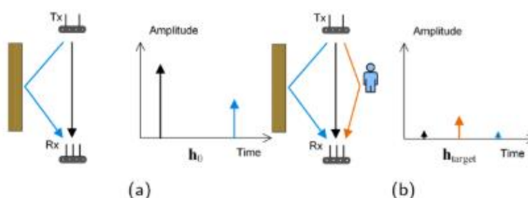
รูปที่ 2.5 แผนภาพช่องสัญญาณพื้นหลัง และช่องสัญญาณเป้าหมายกรณีเป้าหมายก่อให้เกิดพาธสะท้อนเพิ่มเติม [2]
